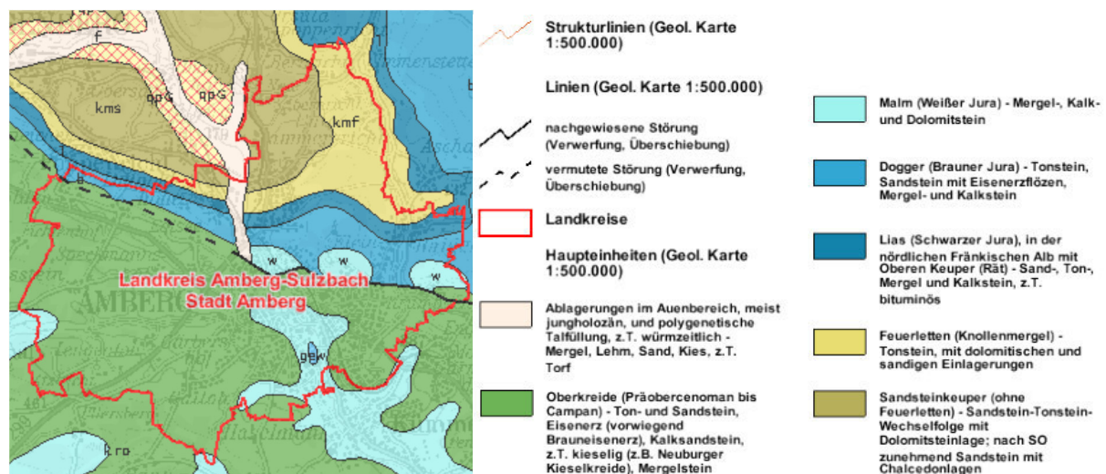
Abb. 3: Geologie
