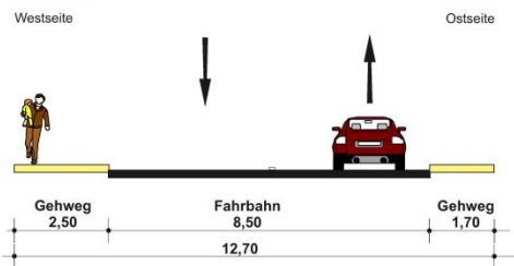
Schlachthausstraße südlich Gasfabrikstraße Bestand
