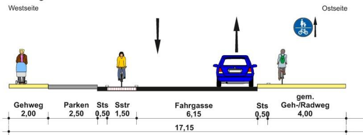
Hirschauer Straße zwischen Akazienweg und Oberammersrichter Weg Lösungsansatz
