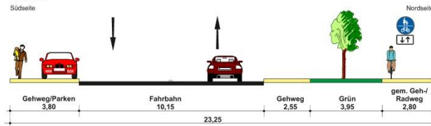
Hockermühlstraße zwischen Wingershofer Straße Bestand
