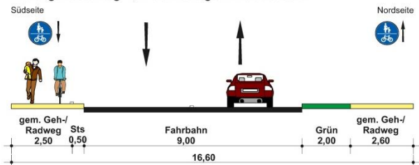
Lösungsvorschlag 1, mit einseitigem Bordversatz
