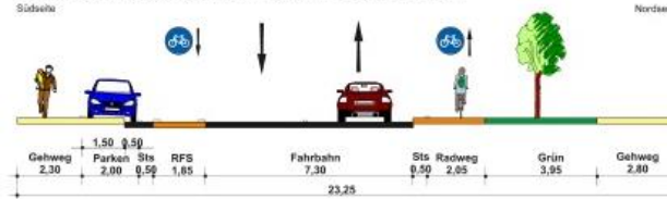
Lösungsvorschlag 2, aufgesetztes Parken und Radfahrstreifen
