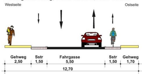
Lösungsvorschlag, Schutzstreifen, ohne Umbau
